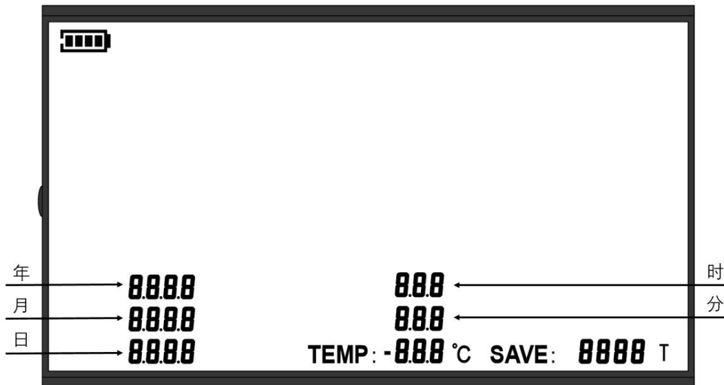
图 14 时钟显示屏幕布局
