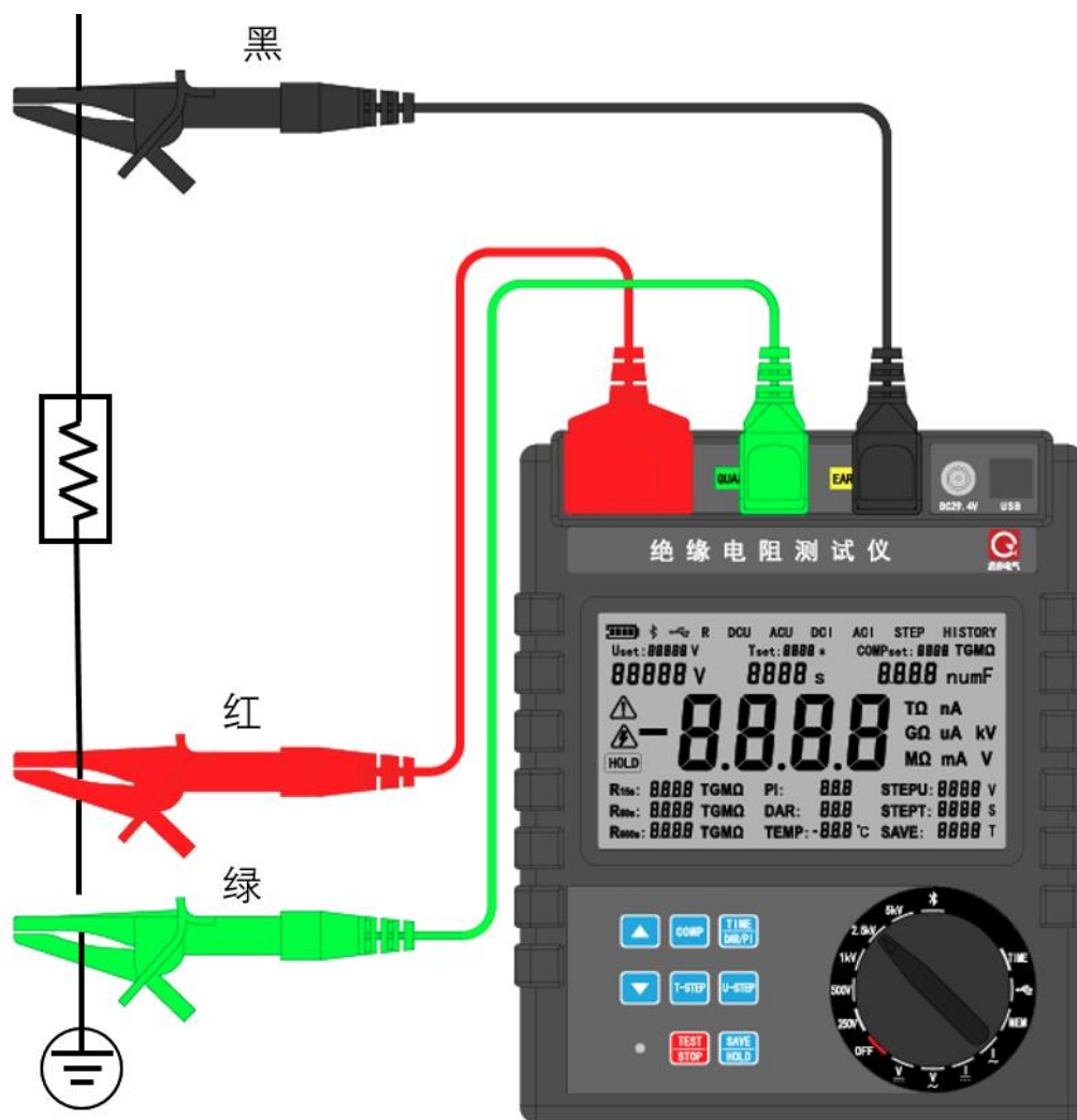
图 8 绝缘电阻测量接线图
