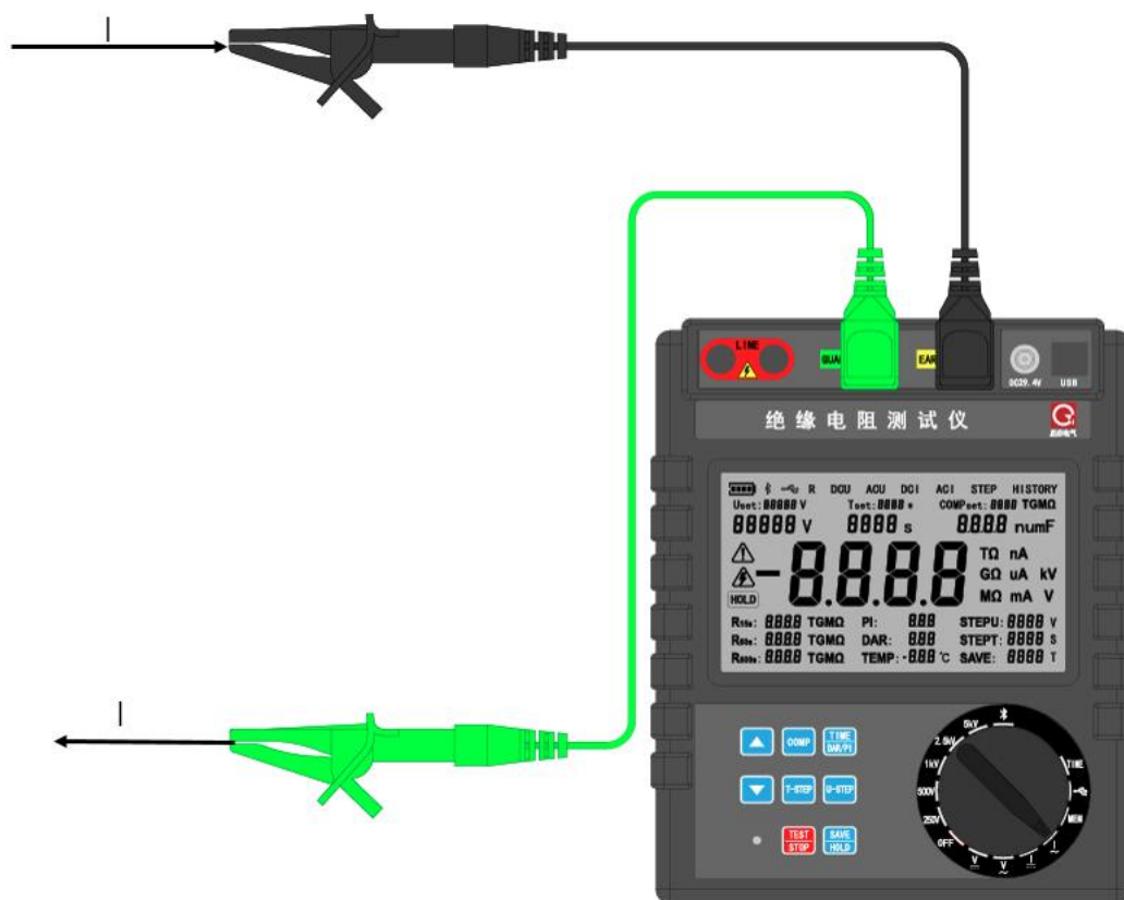
图 13 电流测量接线图
