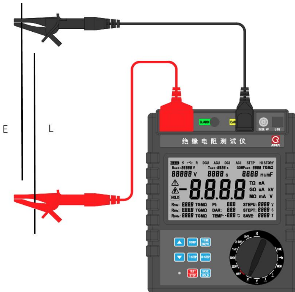
图 12 电压测量接线图
