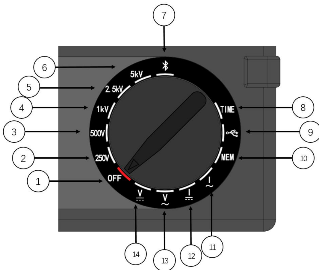
图 6 旋钮档位布局
