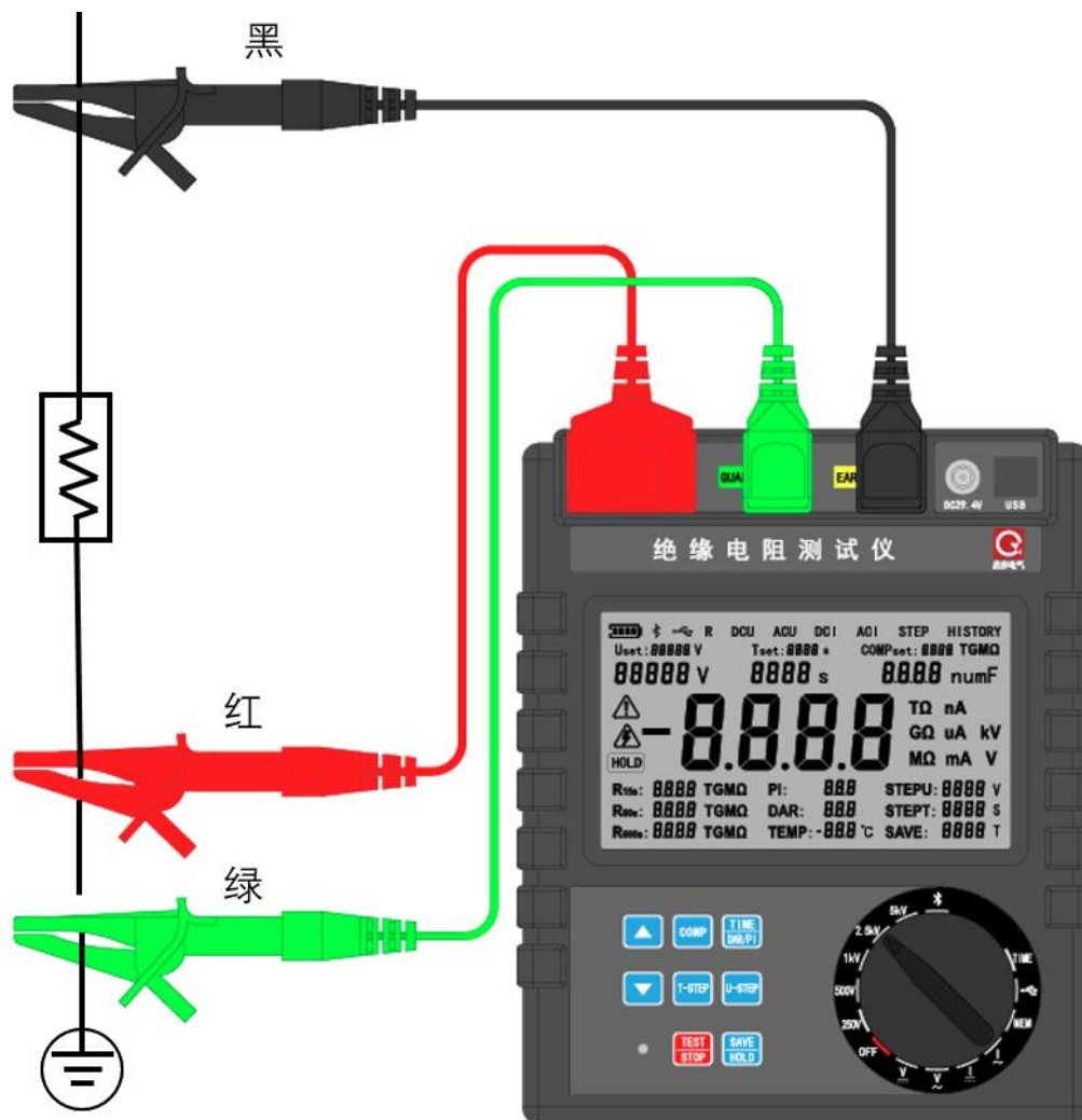
图 7 绝缘电阻测量接线图
