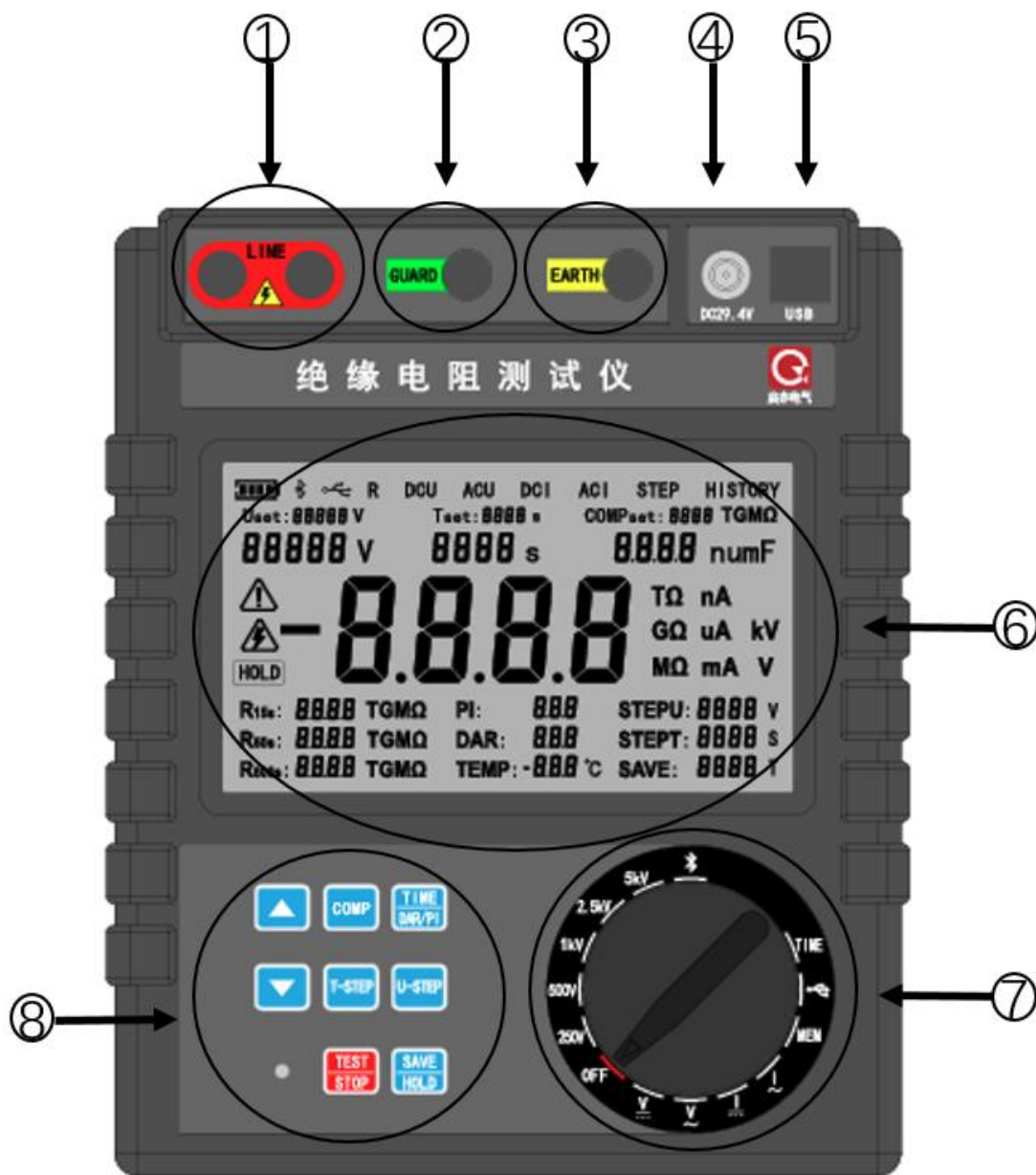
图 3 面板布局图
